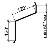
металлический элемент тип 4 (развёртка)
