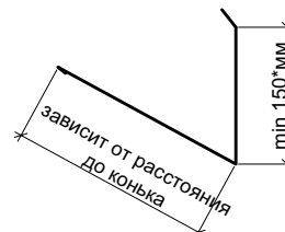
металлический элемент тип 3 (развёртка)
