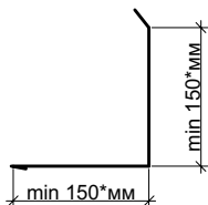
металлический элемент тип 1 (развёртка)
