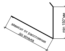
металлический элемент тип 3 (развёртка)
