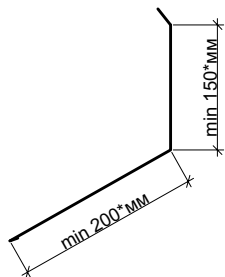
металлический элемент тип 2 (развёртка)
