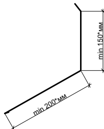
металлический элемент тип 2 (развёртка)
